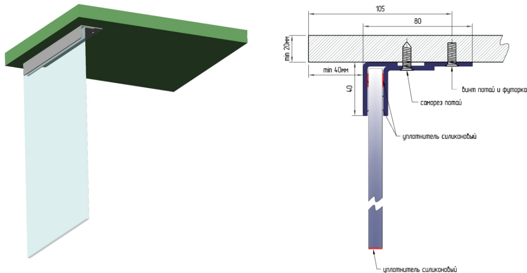
схема расположения крепления
